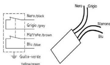
Circuito elettrico microinterruttore con N°2 contatti NC
